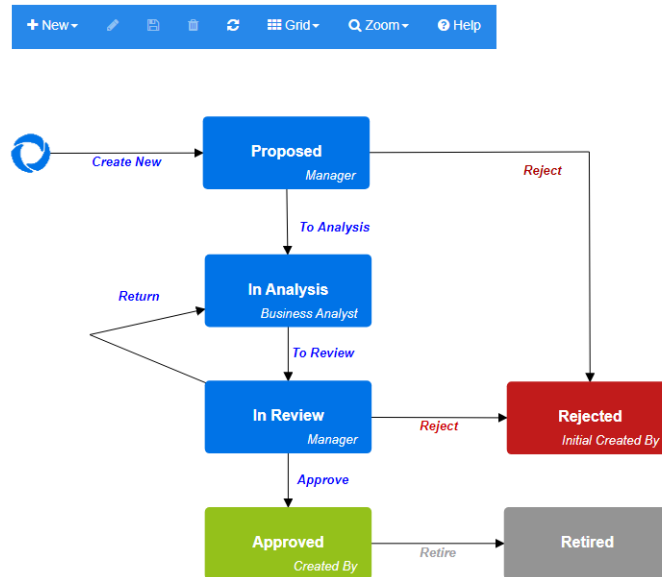
図 11-12. クラス Product_Requirements のワークフロー
