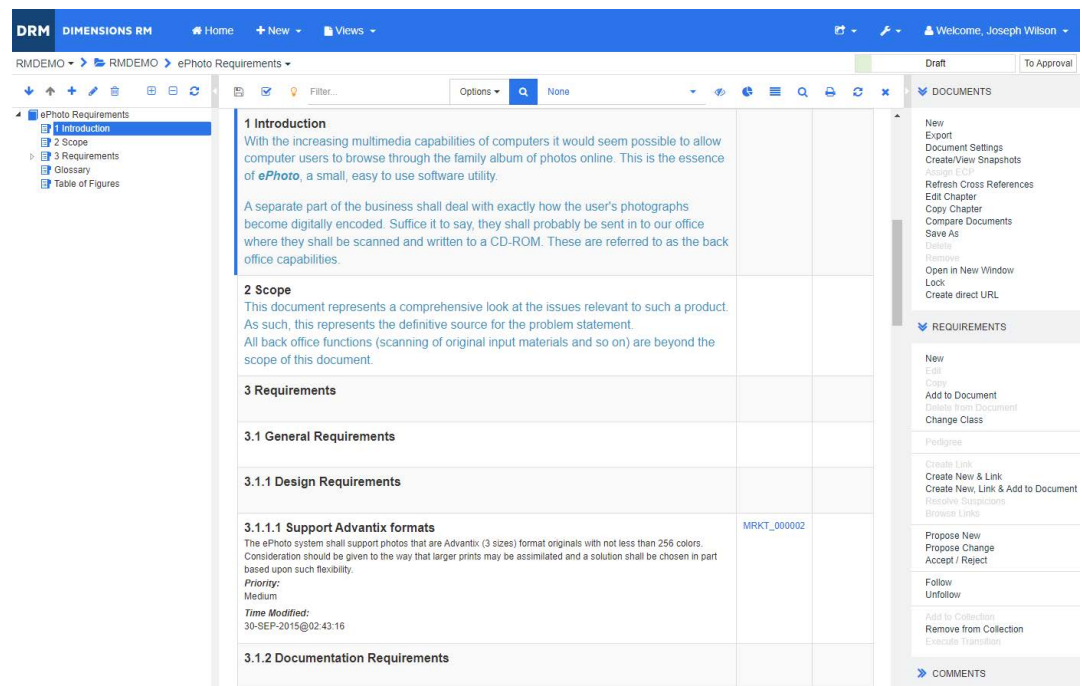
図 4-3. ドキュメントビューモード：ドキュメント全体（コンパクトモード）
