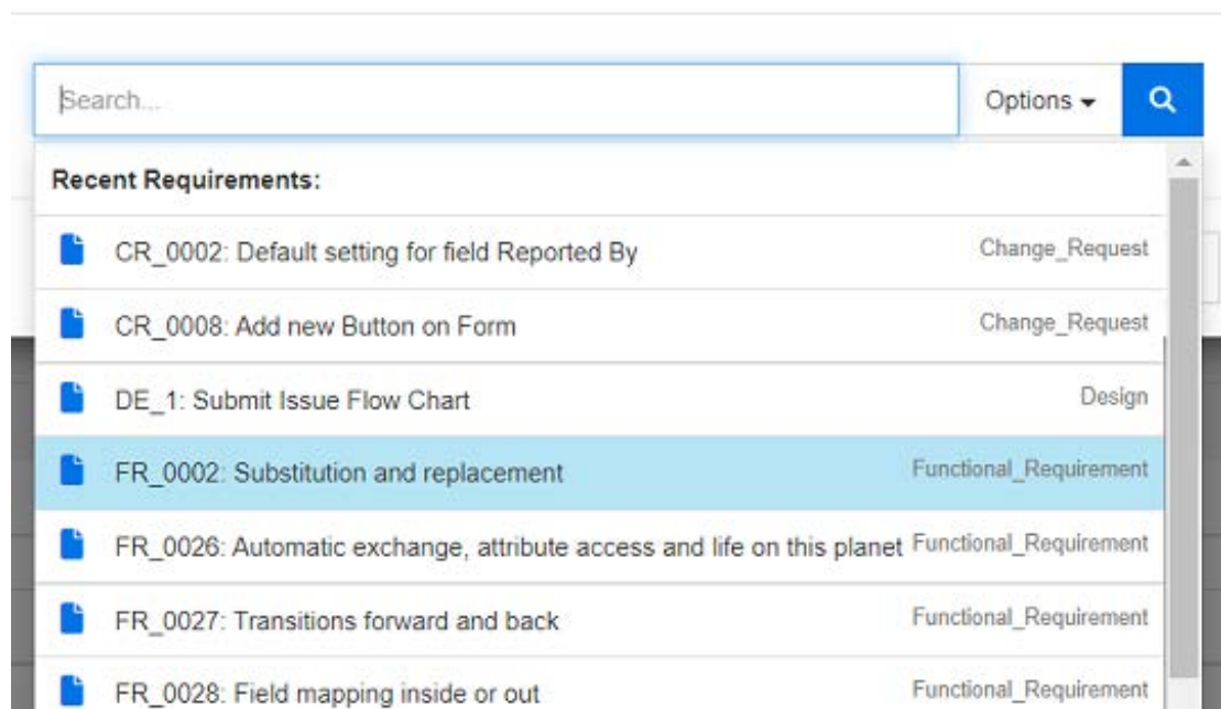
Figure 3-7. Cliquez dans la zone « Rechercher... » pour forcer l'affichage des exigences consultées récemment ou saisissez une chaîne de recherche.
