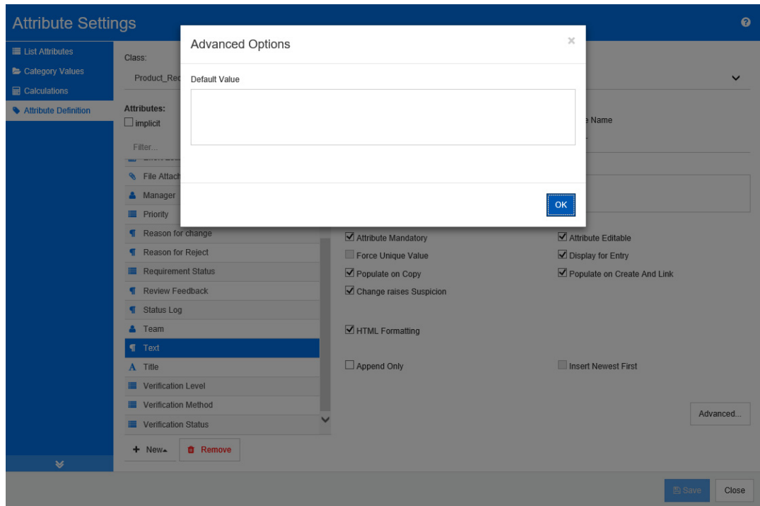
Abbildung 11-8. Textattributdefinition
