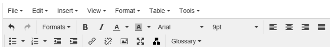
Abbildung 1-1. Standardsymbolleiste "HTML-Textformatierung"
