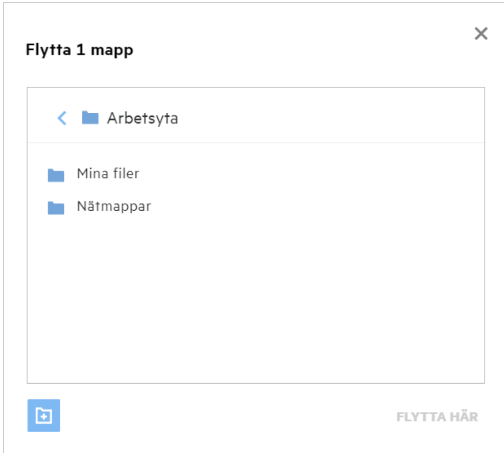
Figure 31 Flytta filer
