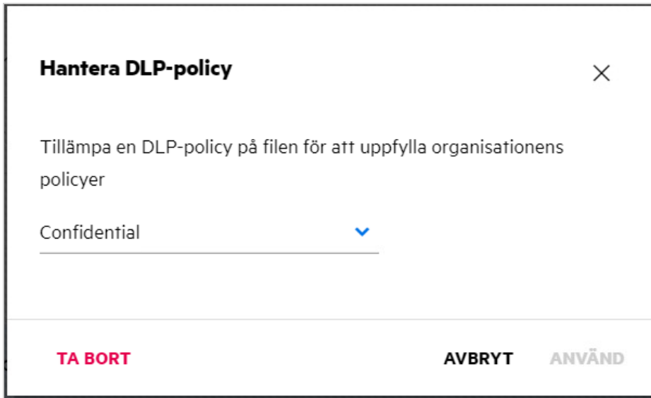
Figure 58 Hantera DLP-princip
