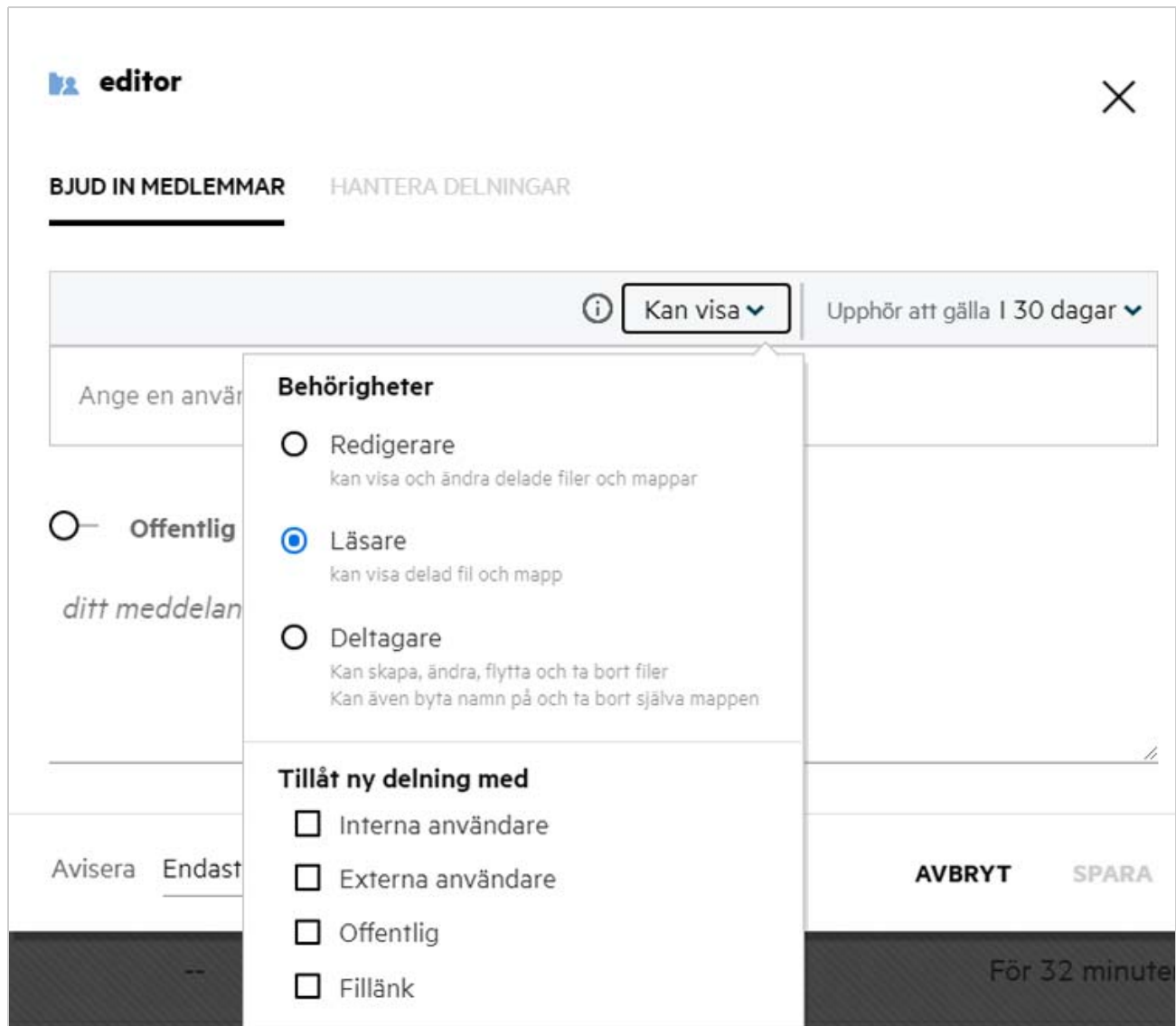
Figure 48 Redigera delningar
