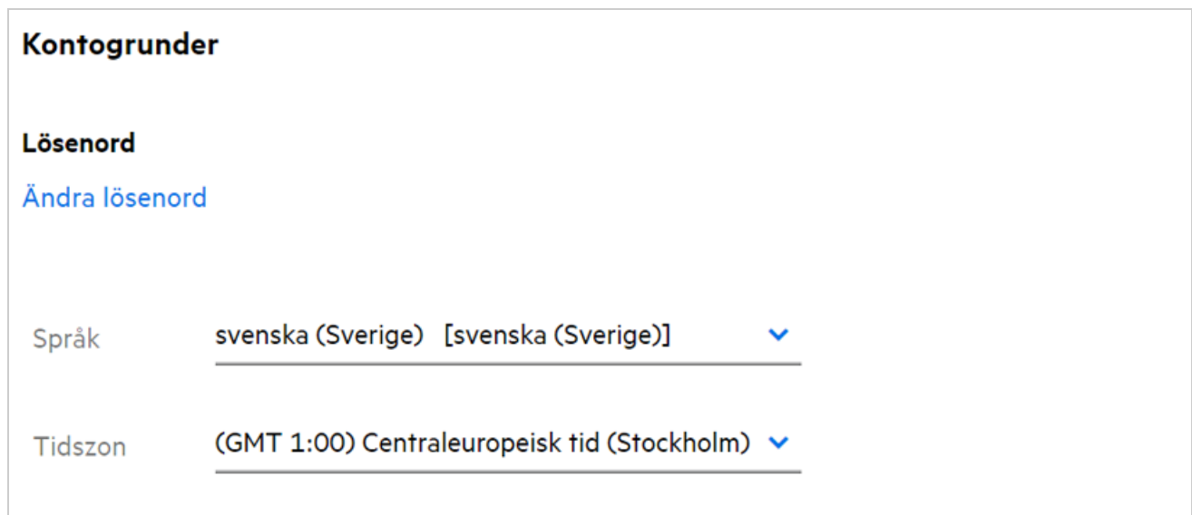
Figure 20 Användarspråk
