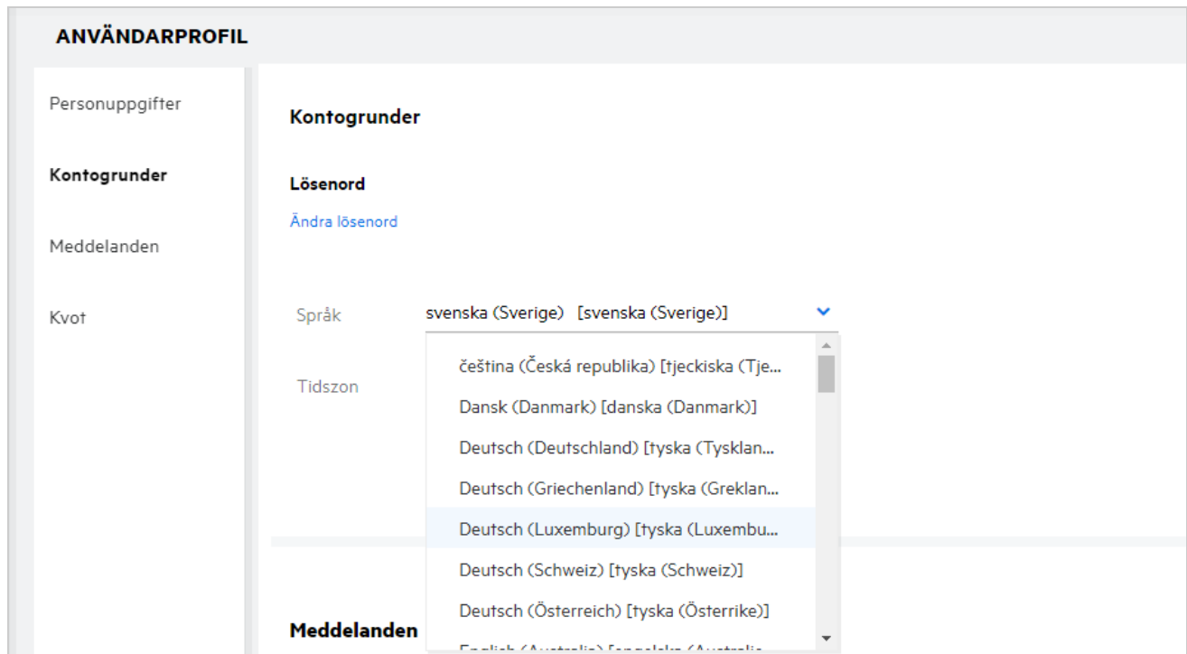
Figure 19 Byt språk
