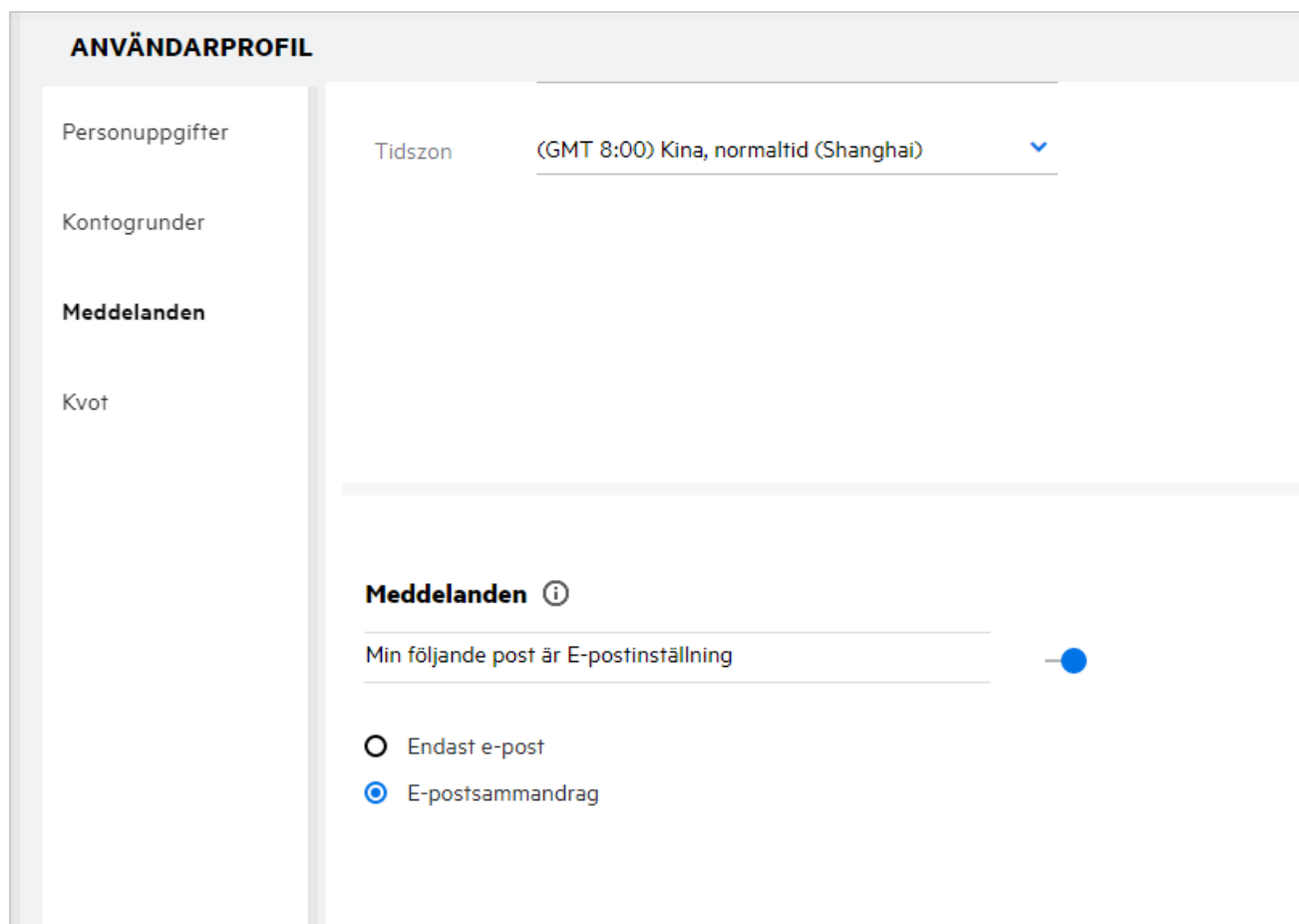
Figure 23 Följaviseringar
