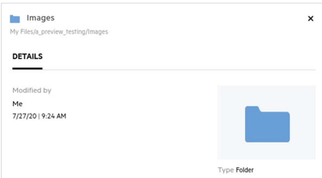
Figure 22 Anglais (États-Unis)
